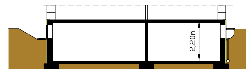
Variante 1: Hochkeller ohne Grundwasser
