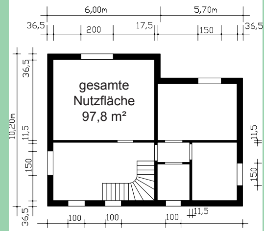
Grundriss des berechneten Kellers
